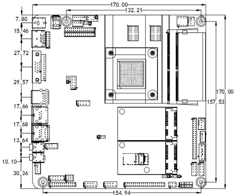
ITX-B413 VER:1.0尺寸图
