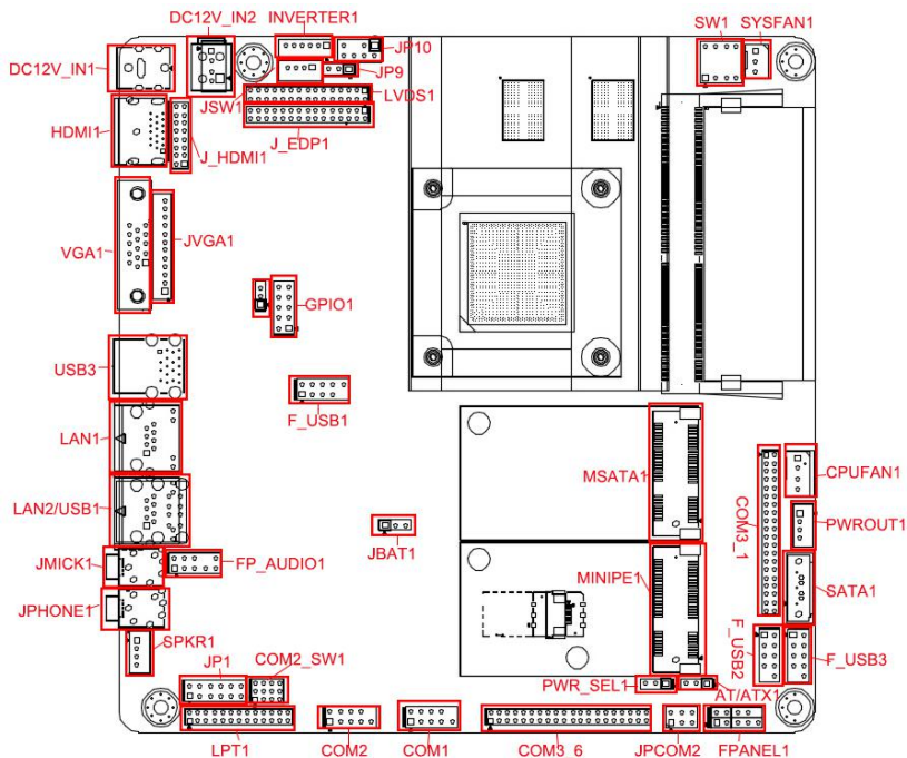
ITX-B413 VER1.0 接口位置图
