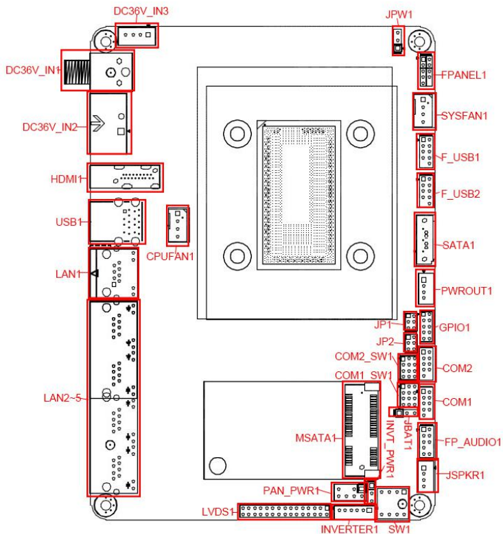
EPIC-W81P4 VER:1.1 接口位置图
