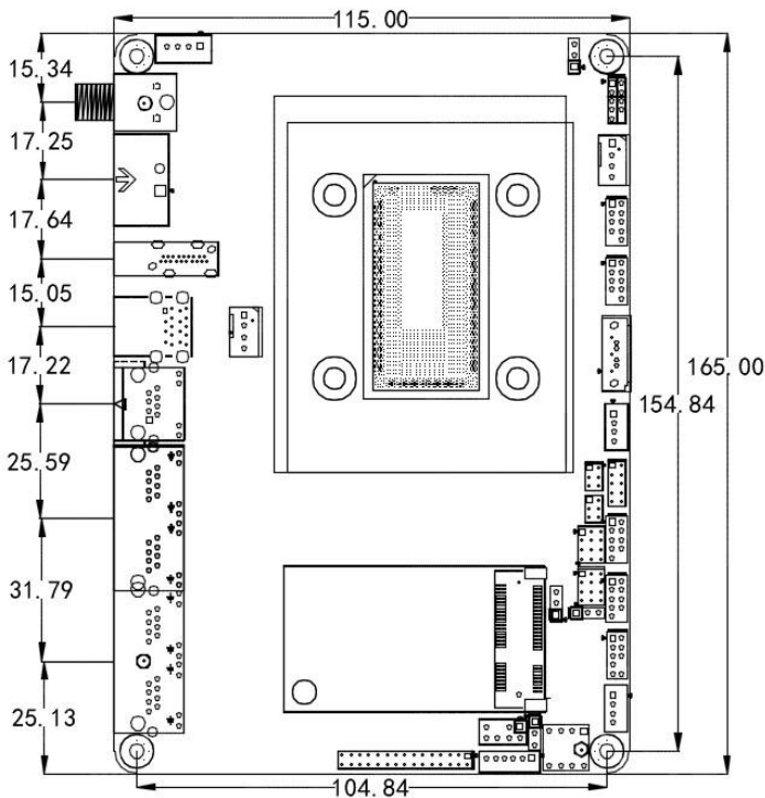
EPIC-W81P4 VER:1.1 尺寸图
