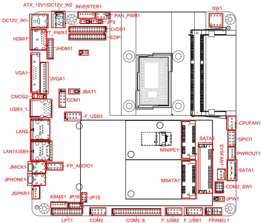
ITX-B430 VER:1.5 接口位置示意图
