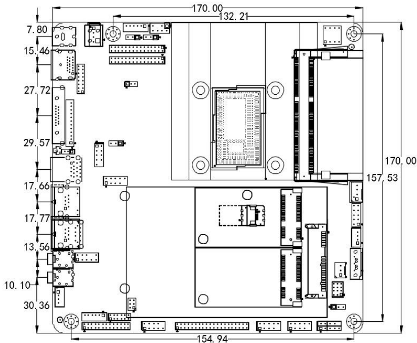
ITX-B430 VER:1.6 尺寸图
