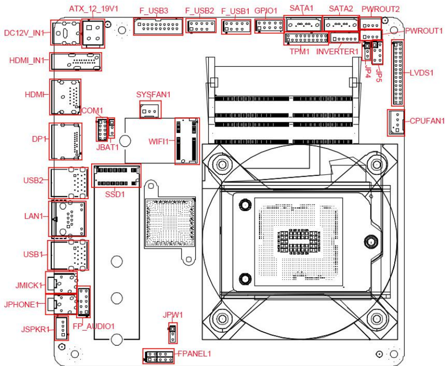
ITX-HW365 VER1.0 接口位置图
