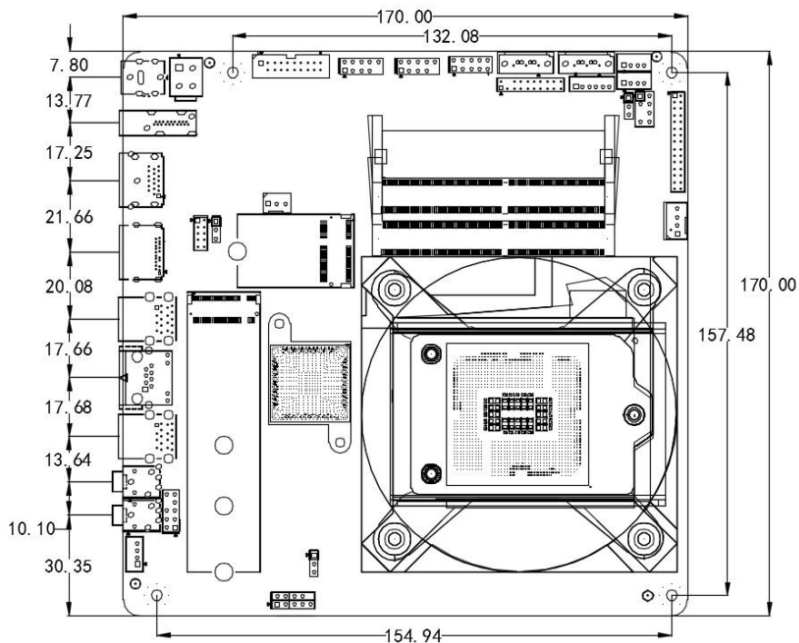
ITX-HW365 VER1.0 尺寸图
