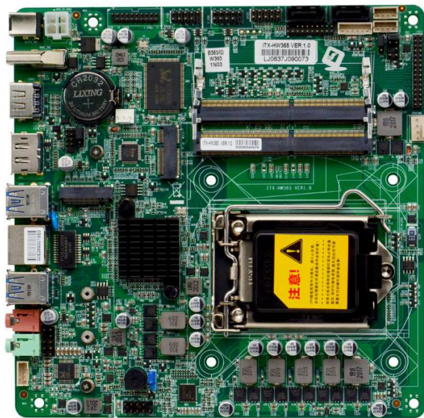
图一：ITX-HW365 VER1.0 正面图
